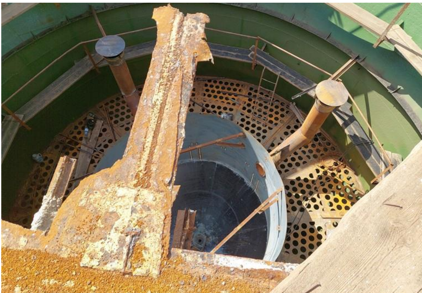
Фото 12 – Монтаж внутренних узлов осветителя
